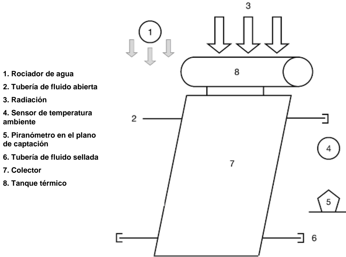
Figura A.5-Choque térmico externo
